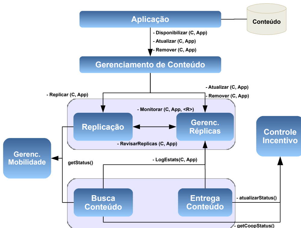
Figura 2. Componentes que devem ser implementados no VCDN. O objetivo é disponibilizar um conteúdo C para alguma aplicação App . Para isso, replicadores <R> são escolhidos para entregar o conteúdo aos interessados.
